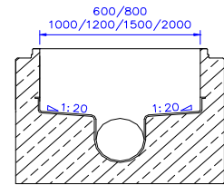
PRECO - Schachtunterteile
